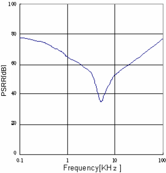
Figure 32. PSRR(Io=0mA)
