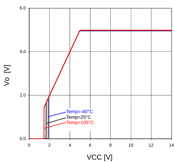
Figure 27. Vcc-Vo ( I_o=0\text{mA} )
