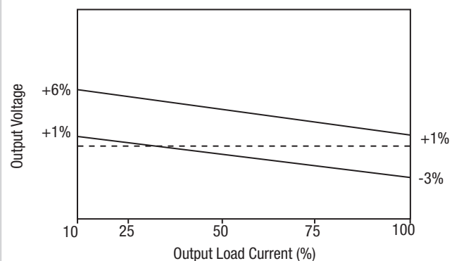
15V Output
