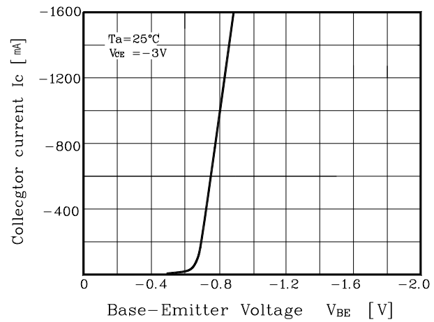
Fig. 2 I_C - V_{BE}
