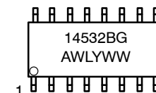
SOIC-16 D SUFFIX CASE 751B
