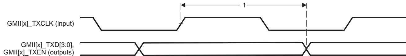
Figure 5-8. GMII[x]_TXD[3:0], GMII[x]_TXEN Timing - MII Mode
