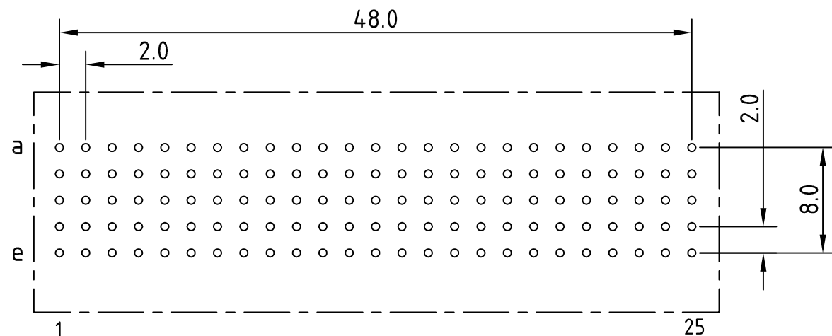
LAY-OUT P.C.B.-HOLE
