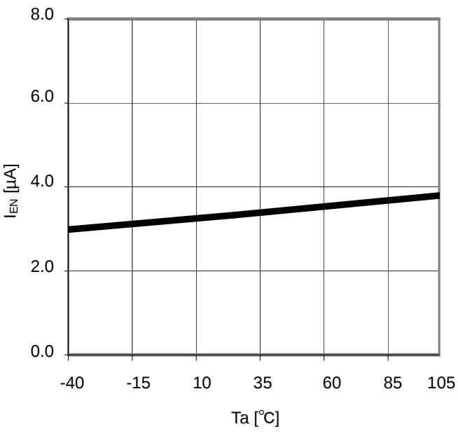
Fig.24 T_a - I_{EN}
