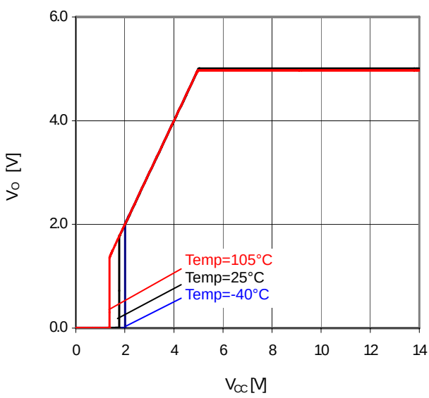
Fig.27 V_{CC}-V_o ( I_o=0\text{mA} )
