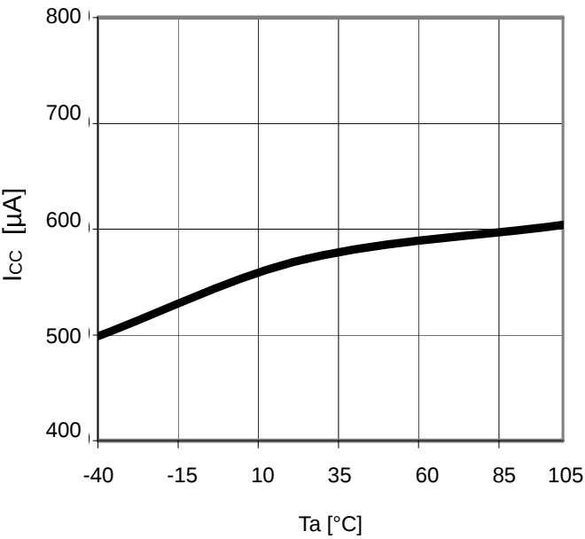
Fig.22 T_a-I_{cc}
