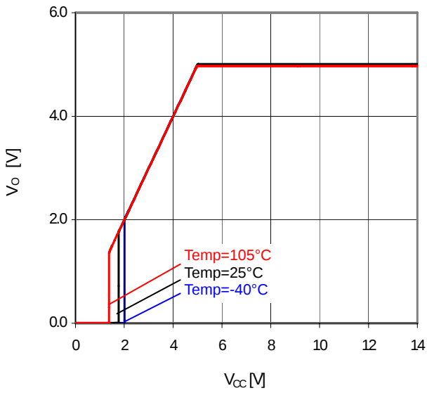
Fig.27 V_{CC}-V_O ( I_O=0mA )
