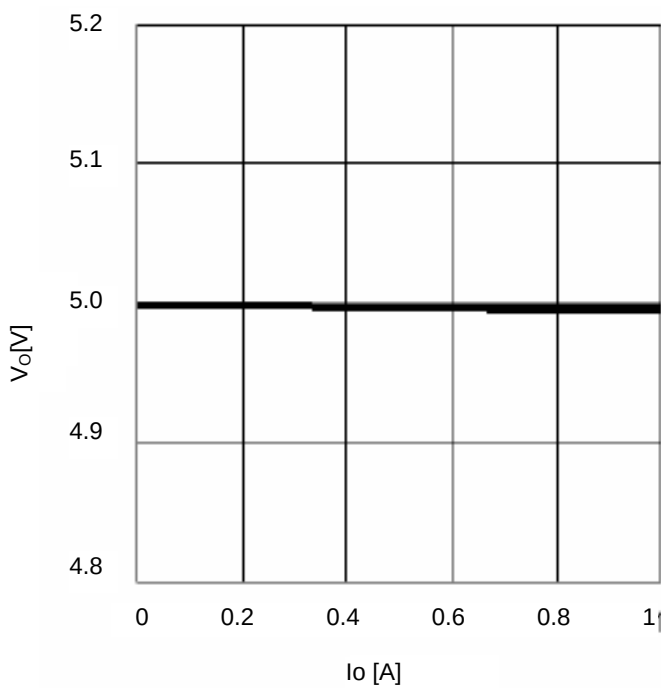
Fig.25 I_O - V_O
