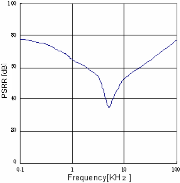
Fig.32 PSRR (Io=0mA)
