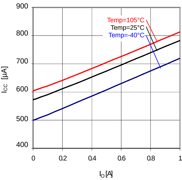
Fig.30 I_o-I_{CC}
