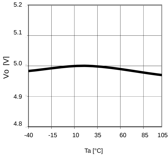
Fig.21 T_a-V_o ( I_o=0\text{mA} )
