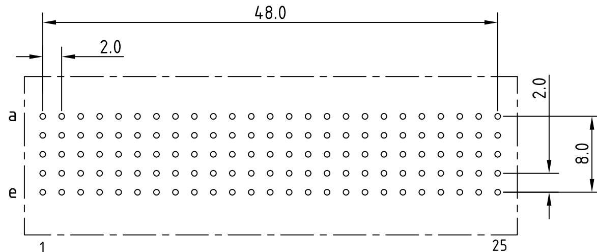
LAY-OUT P.C.B.-HOLE
