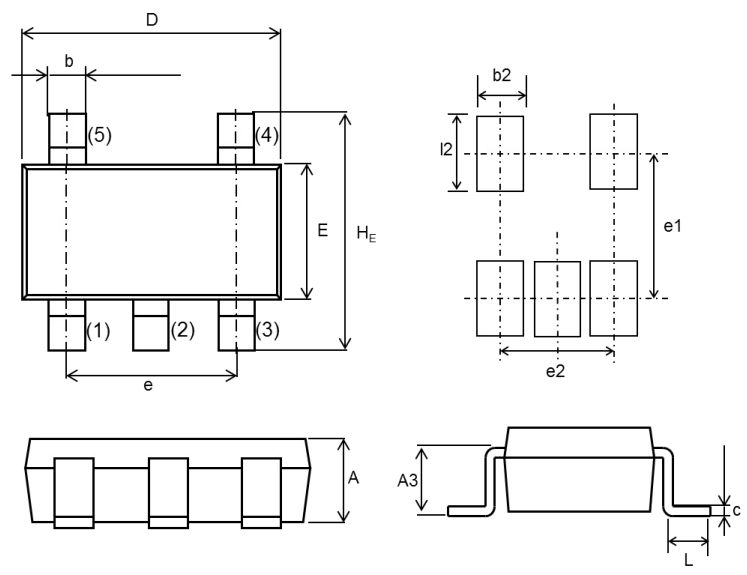
SOT-25T, (TSMD5)
