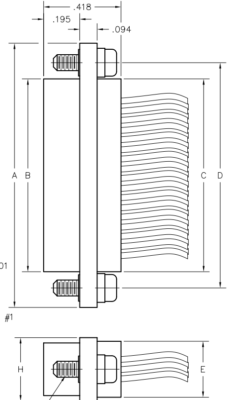
RECEPTACLE
