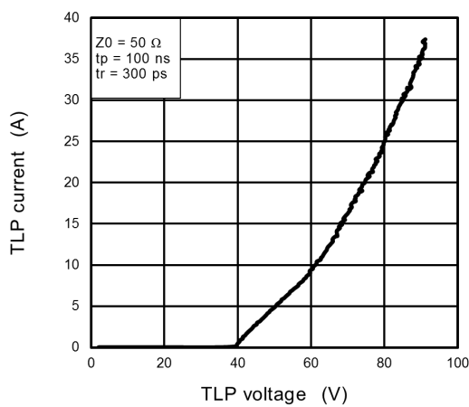
Fig. 9.3 TLP
