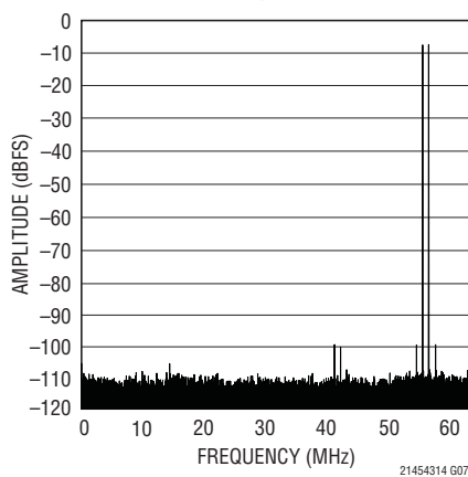
LTC2145-14: 64k Point 2-Tone FFT, f_{IN} = 69\text{MHz} , 70\text{MHz} , -1\text{dBFS} , 125\text{Mps}
