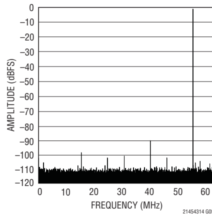
LTC2145-14: 64k Point FFT, f_{IN} = 70\text{MHz} , -1\text{dBFS} , 125\text{Mps}
