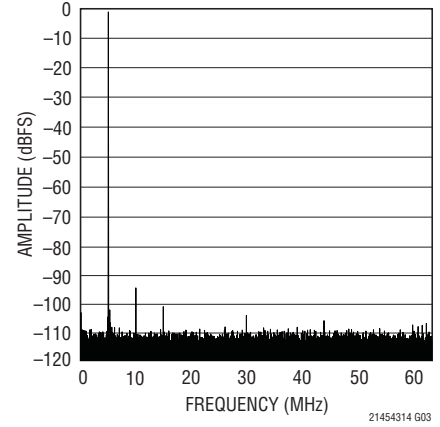
LTC2145-14: 64k Point FFT, f_{IN} = 5\text{MHz} , -1\text{dBFS} , 125\text{Mps}
