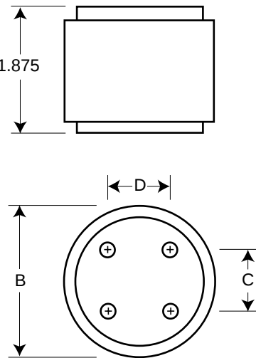
Fig. 2: 4000 Amp Range
