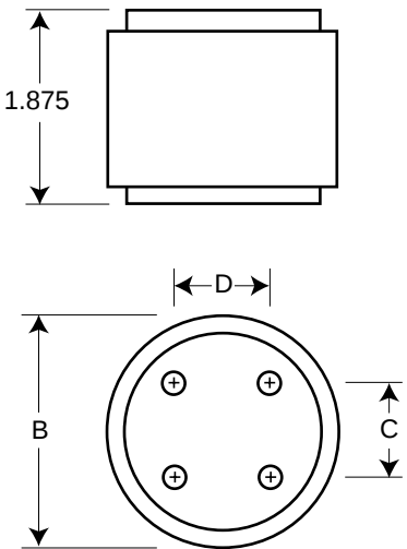
Fig. 2: 4000 Amp Range
