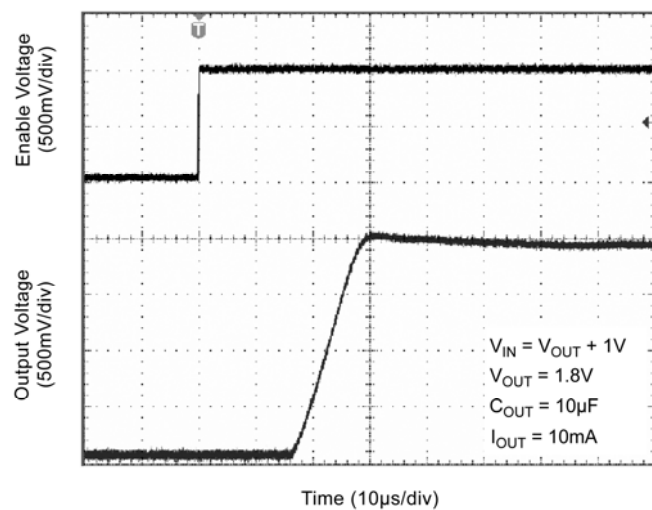
Enable Turn-On
