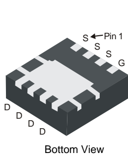
PowerDI3333-8
