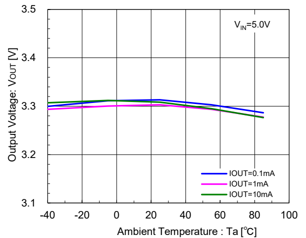
XCL210B331GR-G/XCL210D331GR-G
