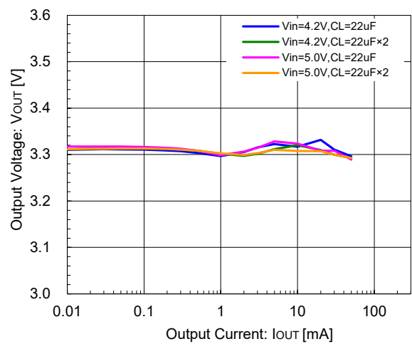
XCL210B331GR-G/XCL210D331GR-G
